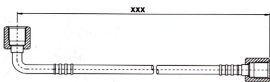
Гибкая капиллярная трубка с прямым фиттингом на 1/4 (SAE) с одной стороны и с угловым фиттингом 90° на 1/4 (SAE) с депрессором
