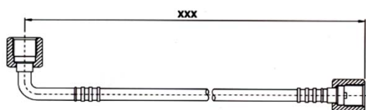
Гибкая капиллярная трубка с угловыми фиттингами 90° на 1/4 (SAE)
