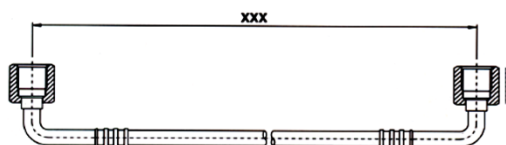
Гибкая капиллярная трубка с угловыми фиттингами 90° на 1/4 (SAE)
