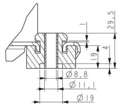
细节A: 压缩机底脚 Detail A: Compressor Foot
